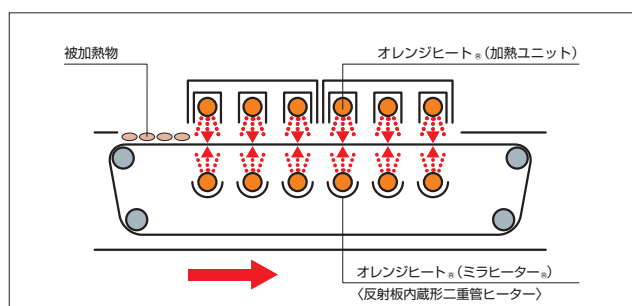
■連続加熱機の構造イメージ図
